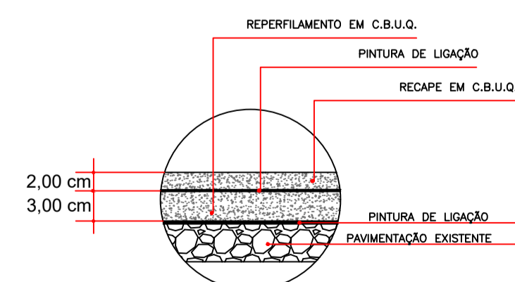
DETALHE RECAPE ASFÁLTICO
